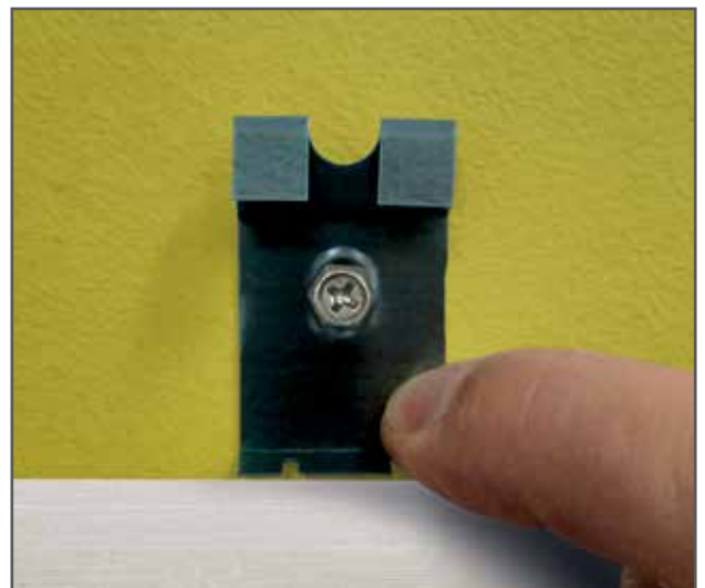
Drugi wariant montażu listwy do ściany: za pomocą uchwyty mocującego. Второй вариант крепления плинтуса к стене: при помощи кронштейна. Another way of mounting the skirting board to the wall: by means of a clamp holder.
